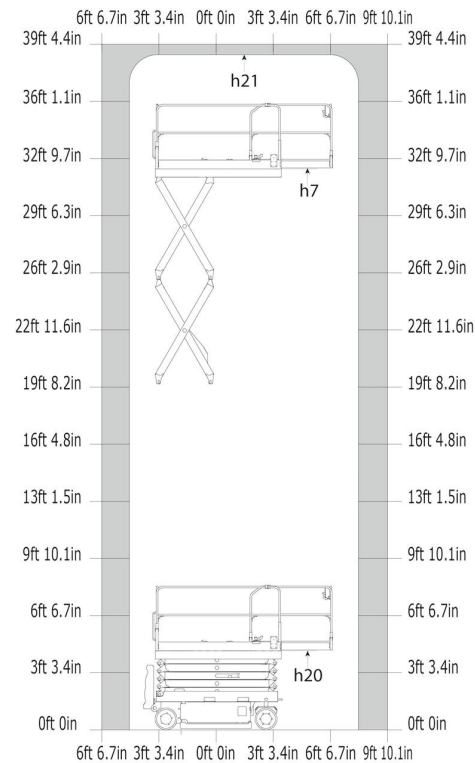
Abaque de charge pour nacelle (impérial)
