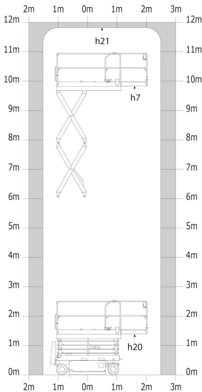
Abaque de charge pour nacelles métrique
