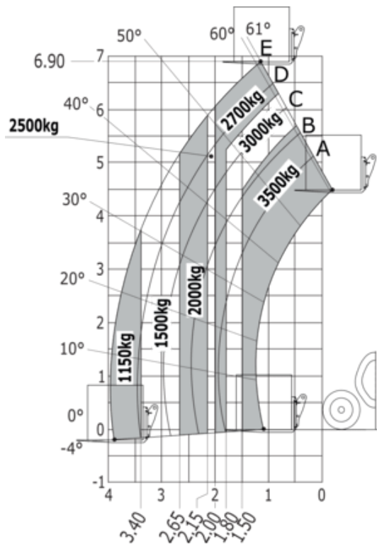
Machine sur pneus avec fourches
