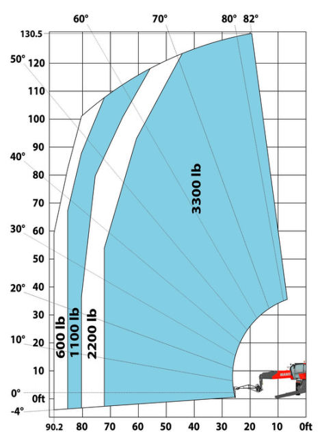
Machine sur stabilisateurs abaissés avec potence-treuil de 1500 kg (Impérial)
