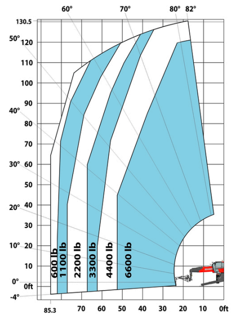
Machine sur stabilisateurs abaissés avec potence-treuil 3000 kg (Impérial)
