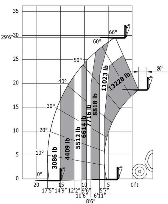
Machine sur pneus avec fourches Impérial
