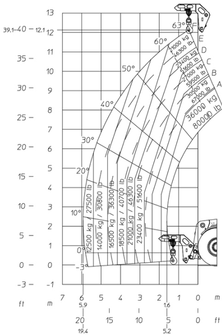
Machine sur pneus avec crochet 36000 kg (Imperial)
