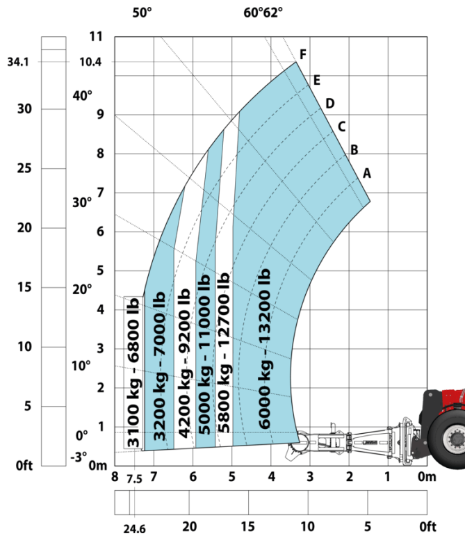
Machine sur pneus avec pince à pneus TH 57 (Métric)
