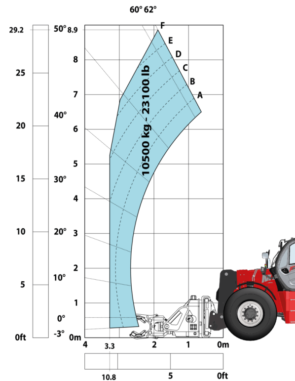
Machine sur pneus avec pince à verins CH 10 (Impérial)
