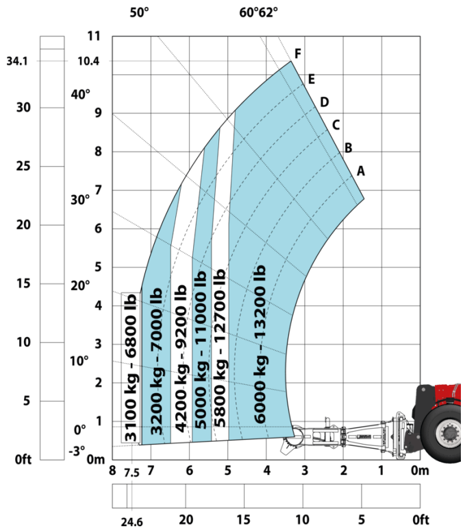
Machine sur pneus avec pince à pneus TH 57 (Impérial)
