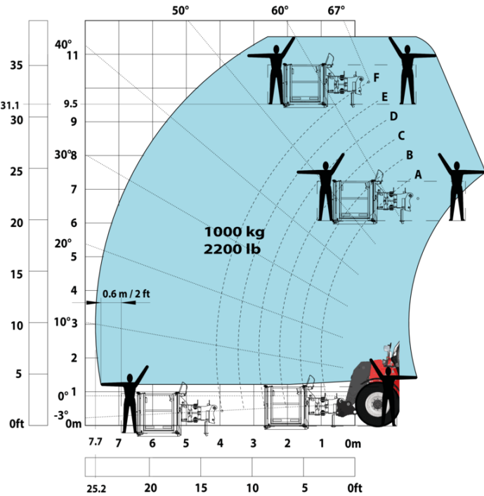
Machine sur pneus avec nacelle Métic
