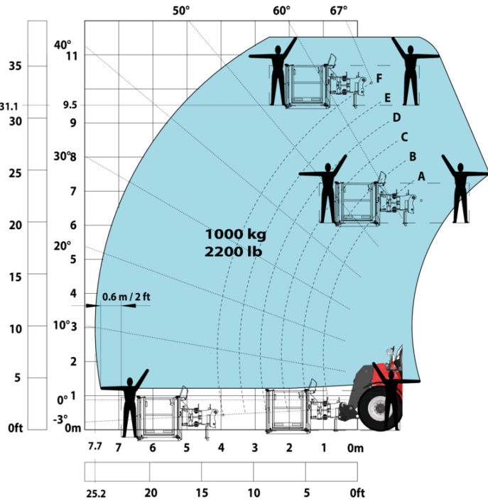
Machine sur pneus avec nacelle Impérial
