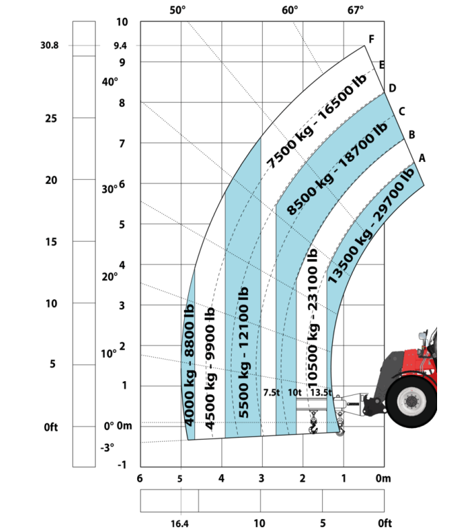
Machine sur pneus avec potence 3 crochets 13500 kg (Imperial)
