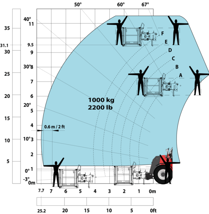
Machine sur pneus avec nacelle Mètric
