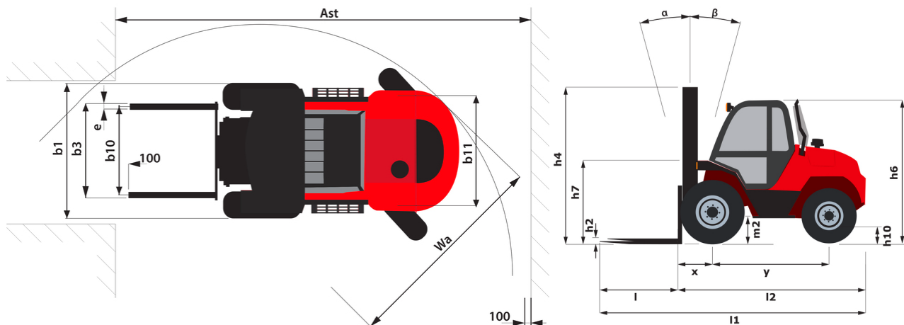
M 40-2 - Schémas d'encombrement
